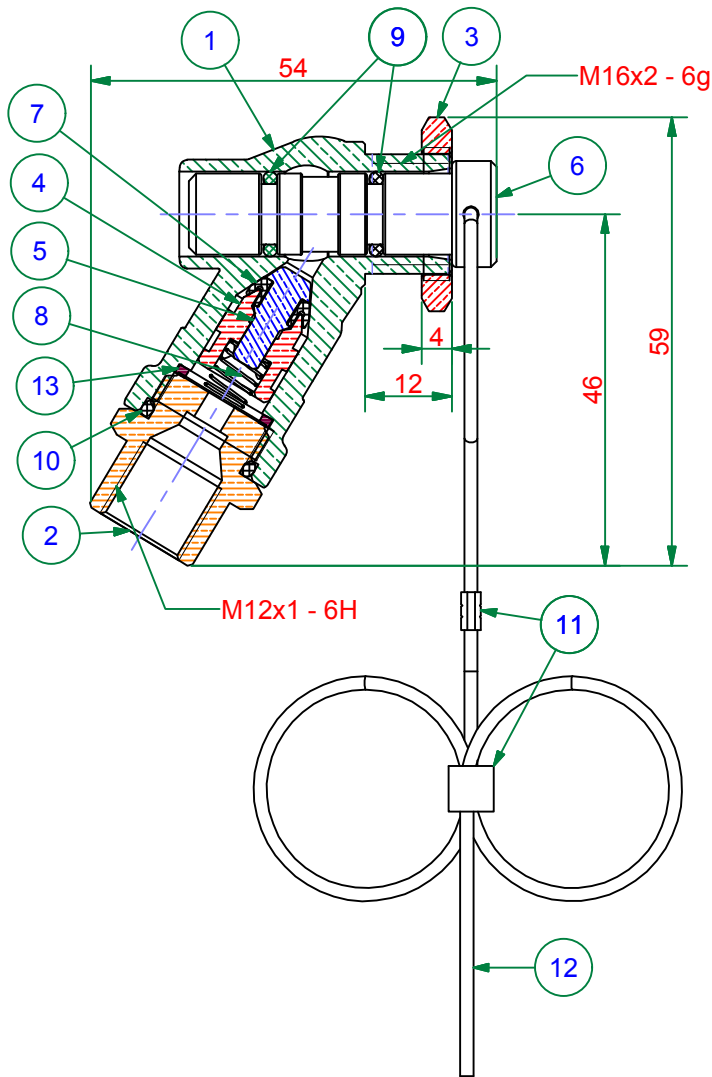
3.4.52.00746 - VÁLVULA GNV ABASTECIMENTO EXTERNO 3.4.52.00746 - CNG EXTERNAL FILLING VALVE
