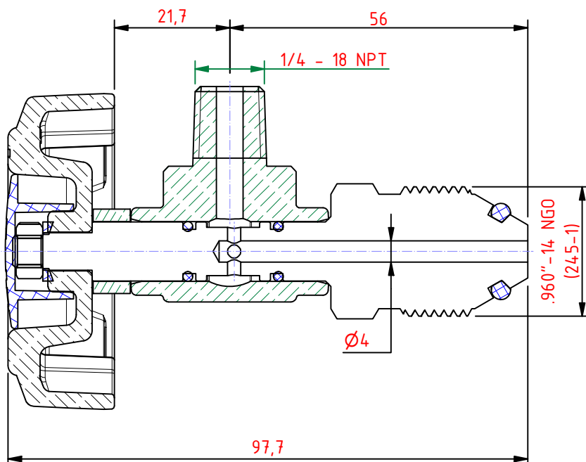
A-A ( 1 : 1 )
