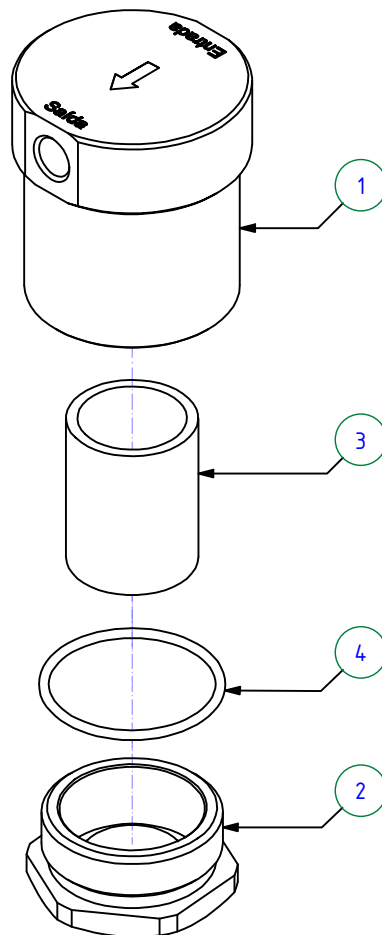
Vista Explodida ( 1 : 2 )
